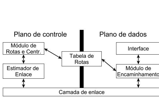
Figura 2. Arquitetura dos algoritmos CRALs.
